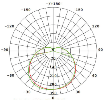
CURVA FOTOMETRICA
